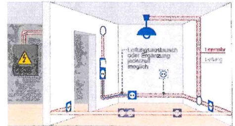
Verlegung von Leerrohring für Steckdosen
